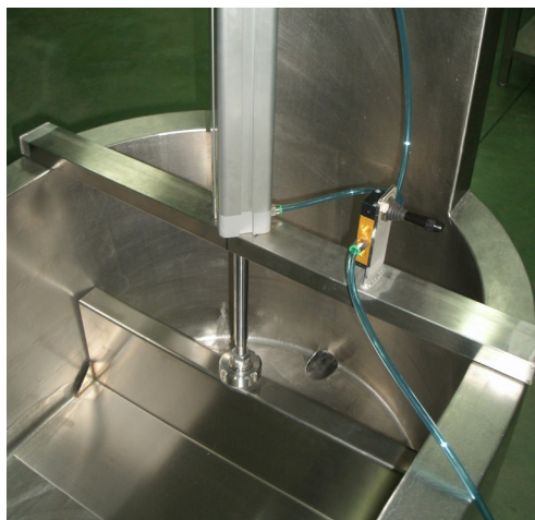
Prototipo mecánico
